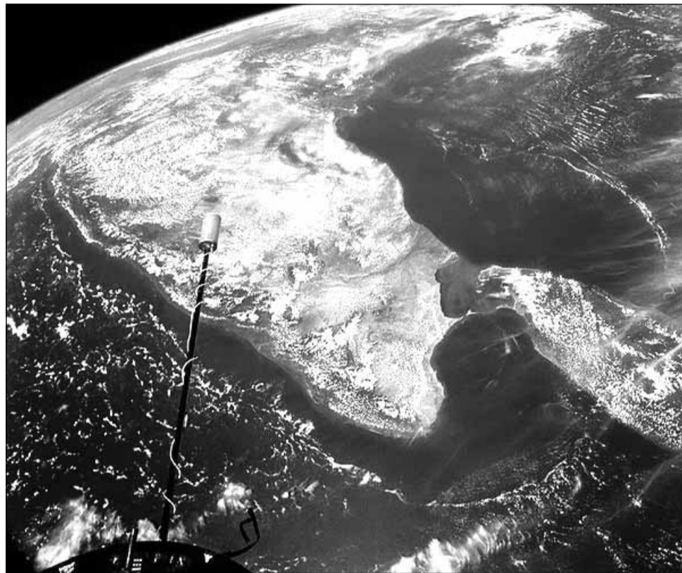
O placă tectonică de dimensiuni impresionante se rupe în două sub Oceanul Indian, într-un timp extrem de scurt... din punct de vedere geologic.
