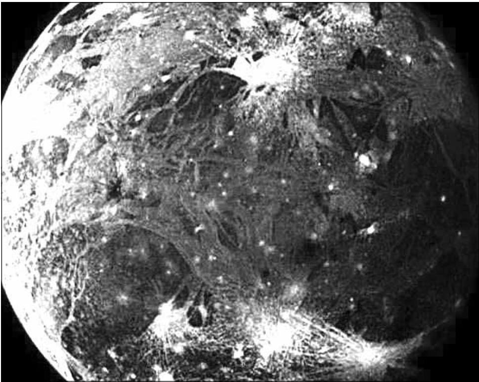
Cel mai mare crater de impact din întregul Sistem Solar acoperă o regiune uriașă de pe cea mai mare lună a lui Jupiter, Ganymede
