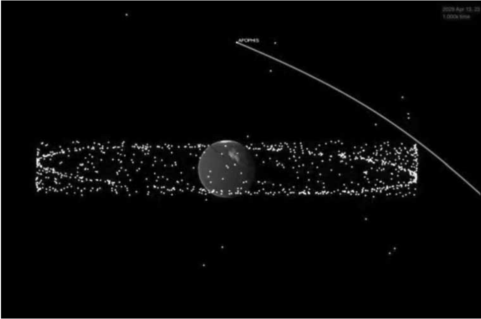
Apophis este un asteroid mare cu o orbită circumsolară aflată în vecinătatea orbitei terestre
